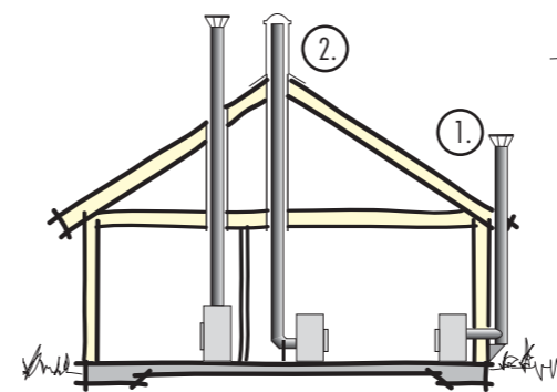
Eksempel på montering med LANDY 2001 DW
