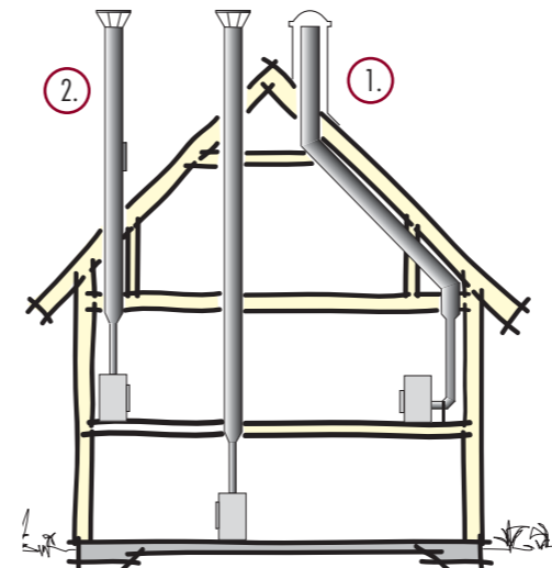
Eksempel på montering med LANDY ROYAL
